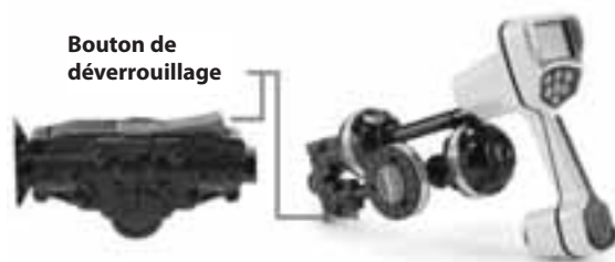
Figure 3: Mât d'antenne pliable et bouton de déverrouillage
