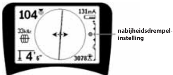
Figuur 33: nabijheidsdrempelinstelling
