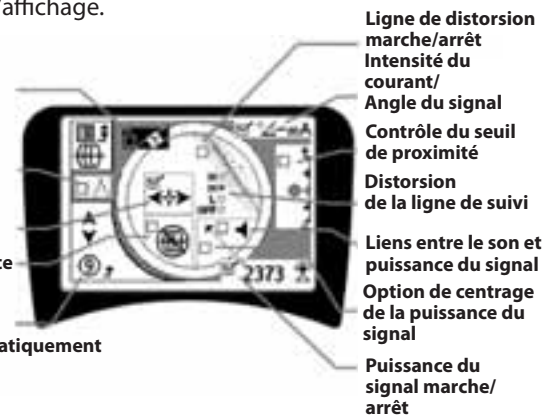
Figure 32: Options d'affichage (Modes Suivi de ligne)
