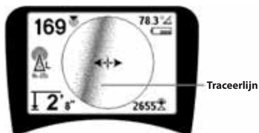
Figuur 20: traceerlijn met veel vervorming
