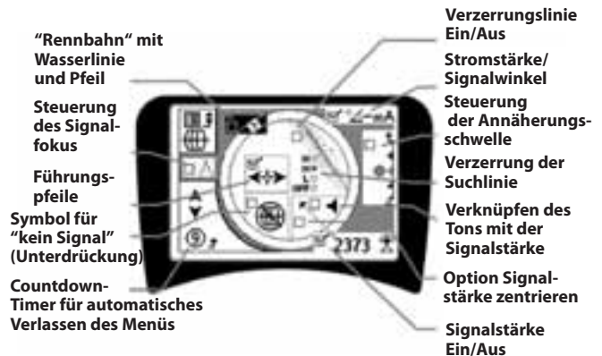
Abbildung 32: Bildschirmelemente (Leitungslokalisierungsmodus)
