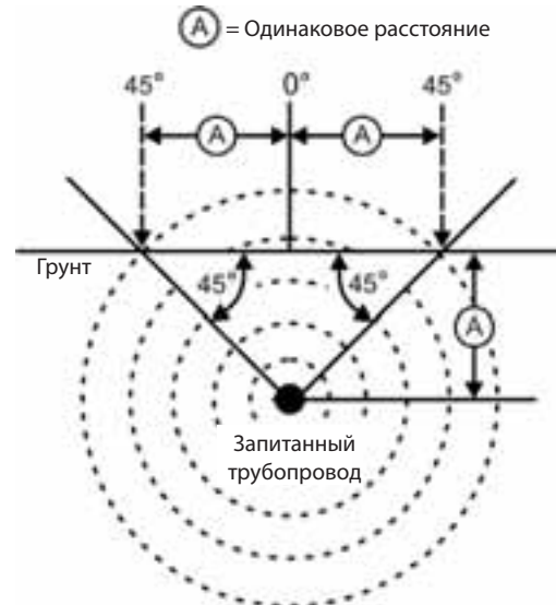
Рис. 22: Проверка искажения
