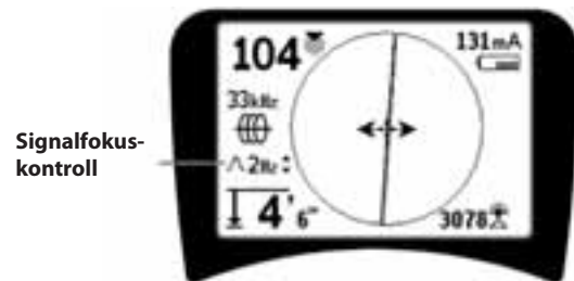
Figur 34: Signalfokuskontroll
