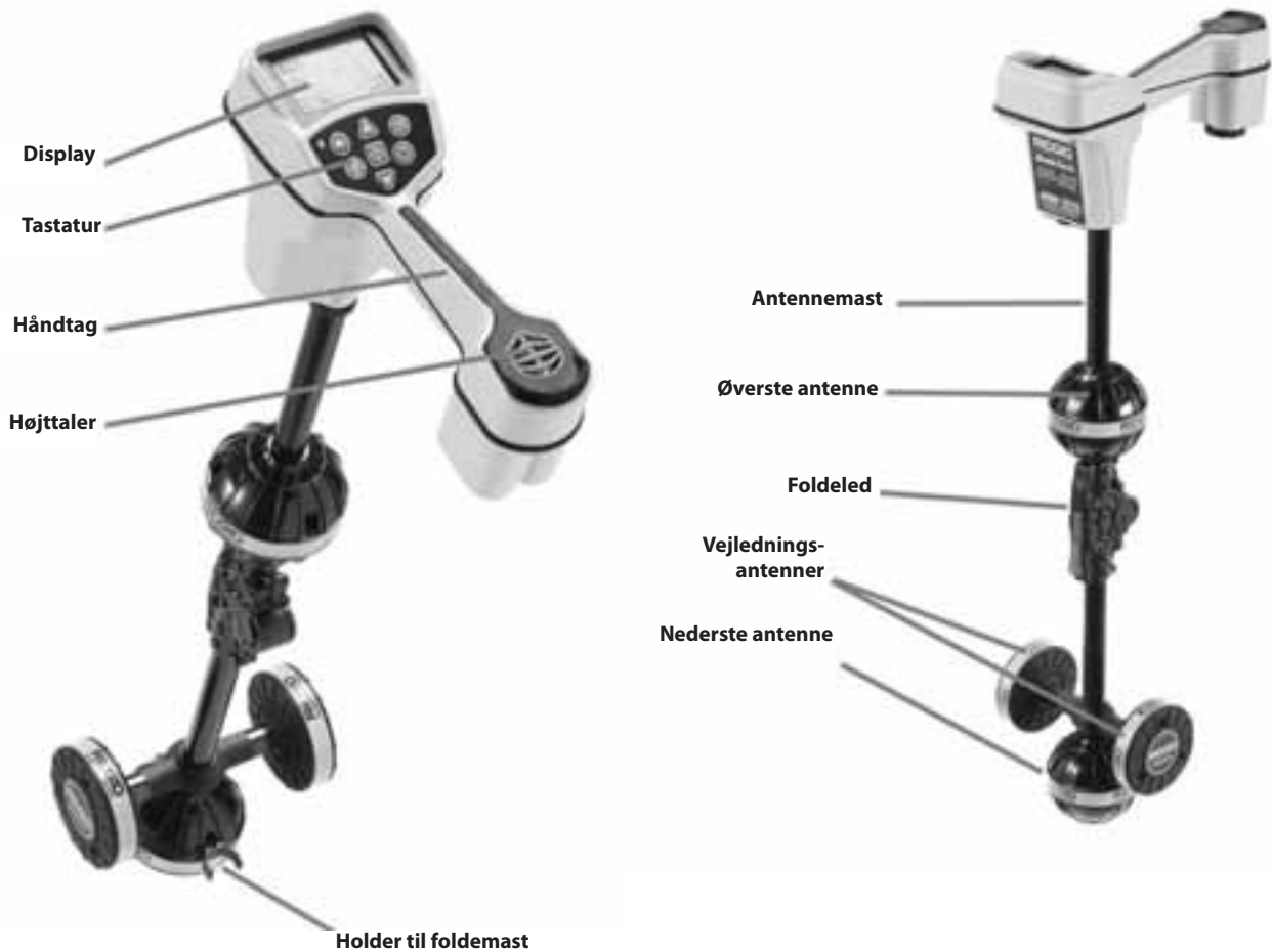
Fig. 1: SR-20-komponenter
