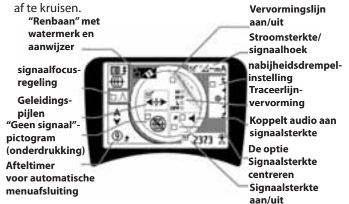
Figuur 32: schermelementen (actieve leidingtracing)
