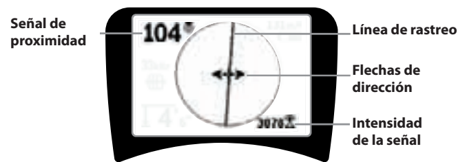
Figura 5: Elementos de pantalla (modo rastreo de línea)
