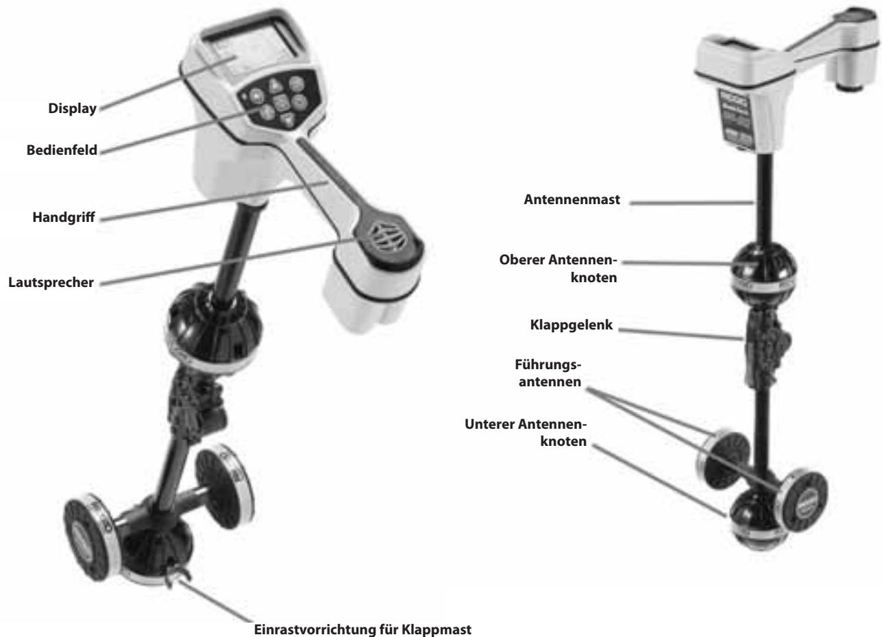
Abbildung 1: SR-20 Komponenten
