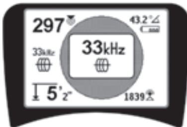
Abbildung 11: Leitungssuchfrequenz Auswahl mit Frequenztaaste
