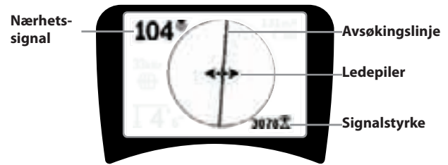
Figur 5: Skjermelementer (linjeavsøkingsmodus)
