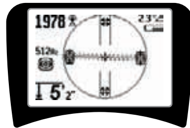
Abbildung 28: Sondenlokalisierung: Äquator
