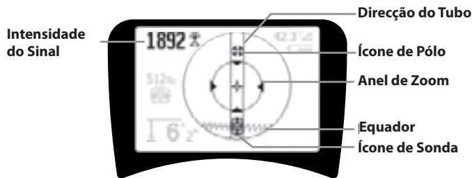
Figura 6: Elementos do Visor: Modo de Sonda
