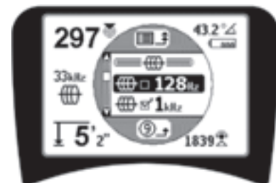
Rysunek 14: Wyróżnianie żadanej częstotliwości (128 Hz)
